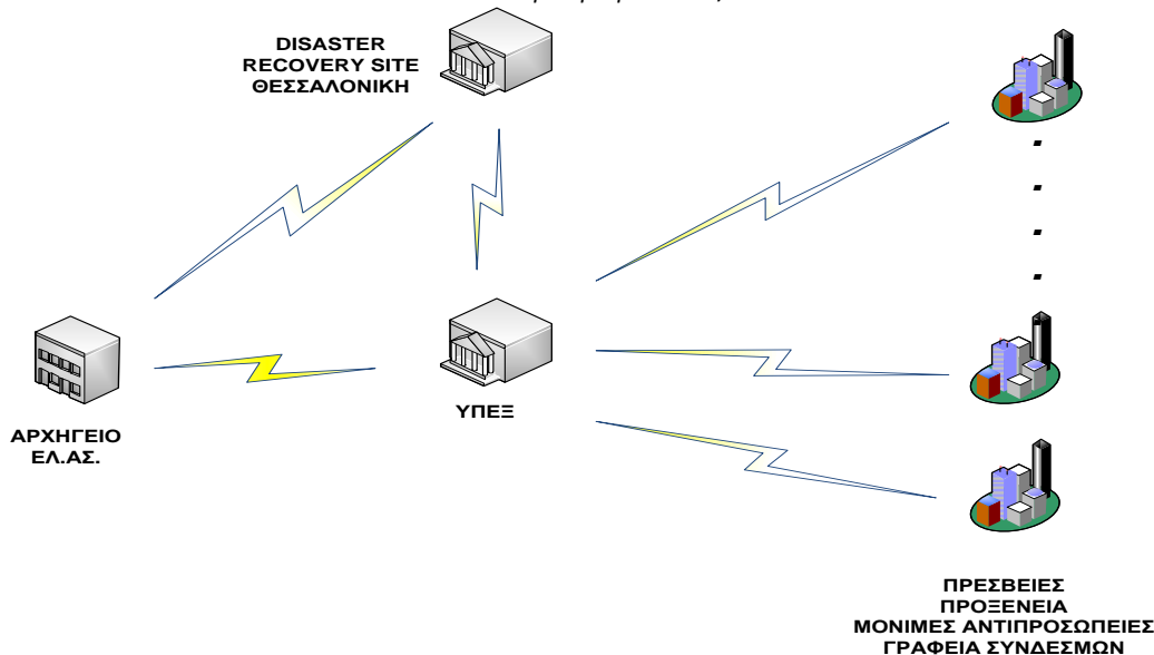
Εικόνα 1: Αρχιτεκτονική Δικτύου NET-VIS
